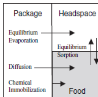
Diagrama de interacción envase – producto.
