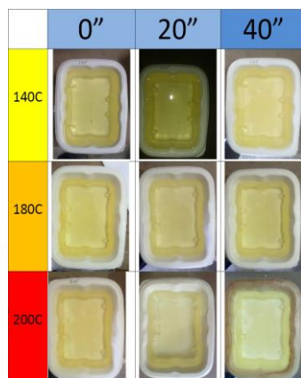
Test estanqueidad a la grasa.
